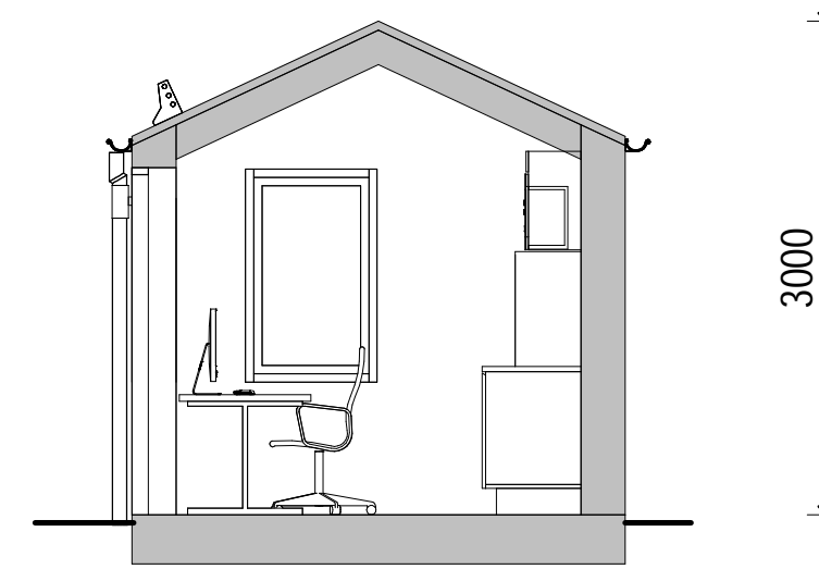
SEKTION A-A
